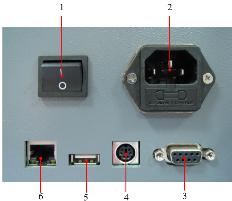
1: Síťový vypínač
